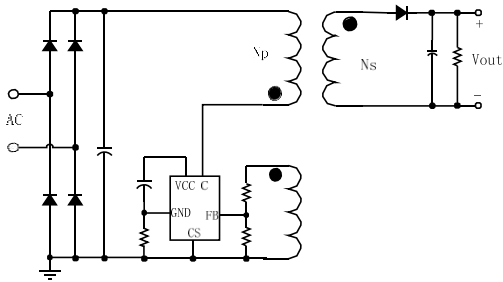
图 1 三绕组典型应用
