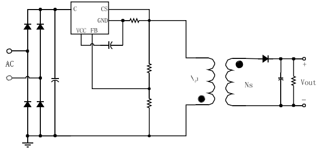
图 2 两绕组典型应用
