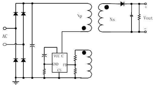
图 1 三绕组典型应用
