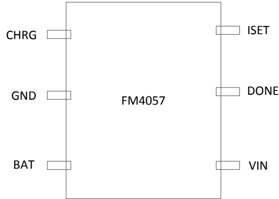
FM4057 引脚图（顶视图）
