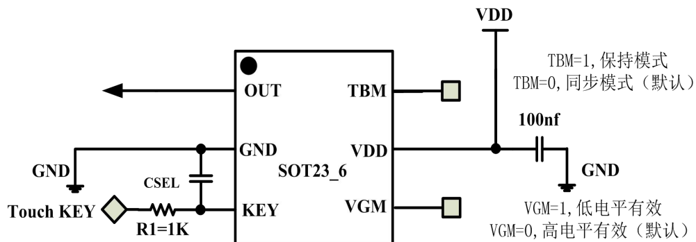
233 应用原理图
