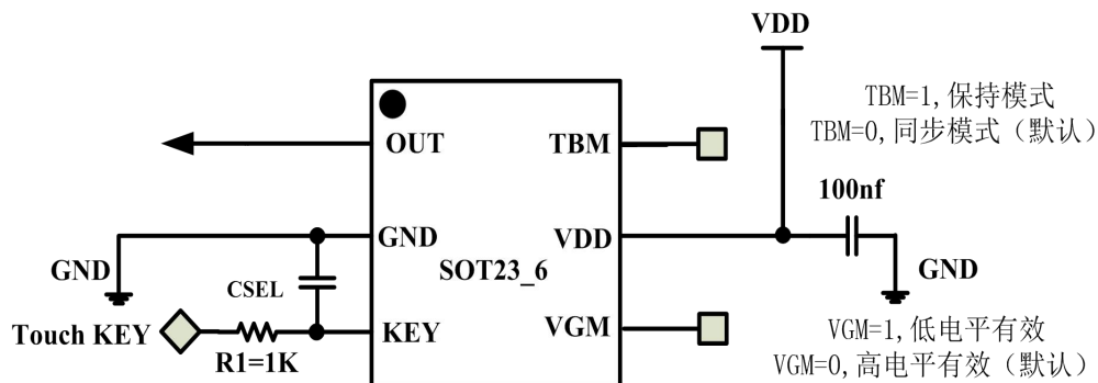
233B 应用原理图
